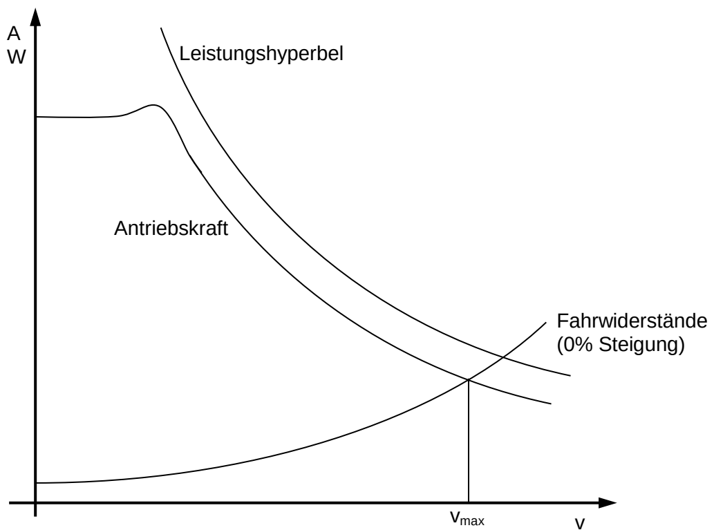
Abbildung: Fahrzustandsdiagramm für einen stufenlosen Automaten.
