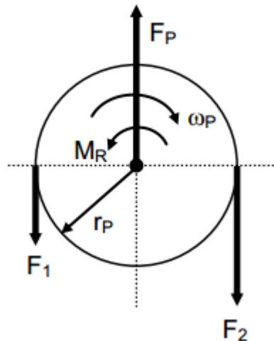
Abbildung: Kräfte und Momente am Planet des Treibachsdifferenzials.
