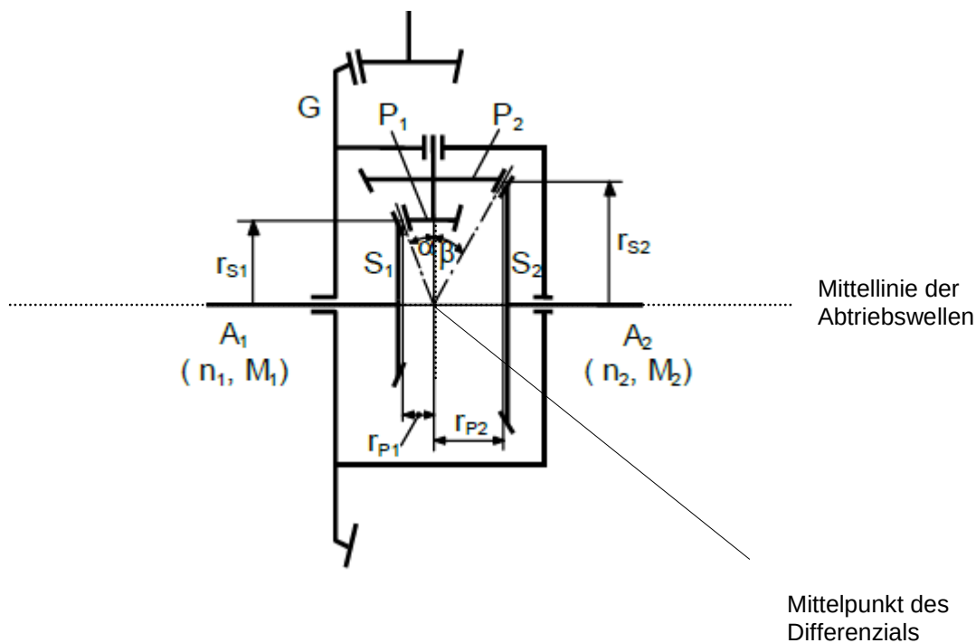
Abbildung: Prinzipskizze zum Verteilerdifferenzial
